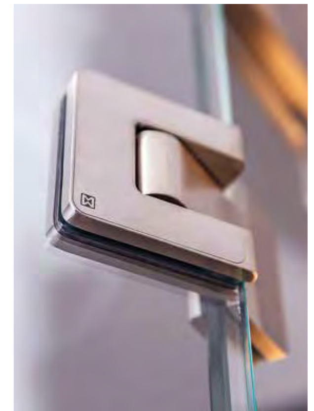
Pendeltürband Agitus L mit Glasanbindung Agitus L swing door hinge, mounted on glass
